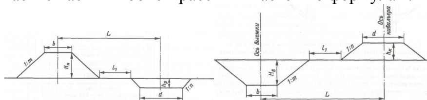
Рис. 4 Поперечный разрез насыпи, отсыпаемой из резерва:
