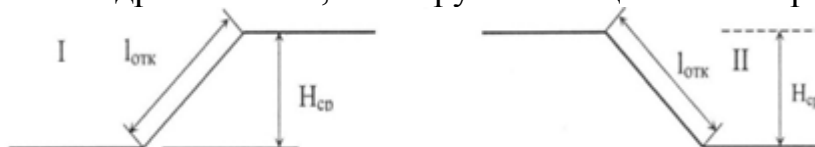
Рис 10 Расчёт длины откоса: I - насыпь; II - выемка.
