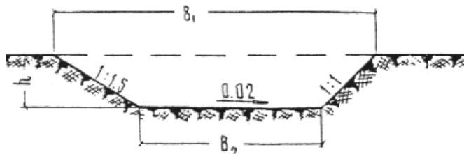
Рис.11 Односкатный резерв
