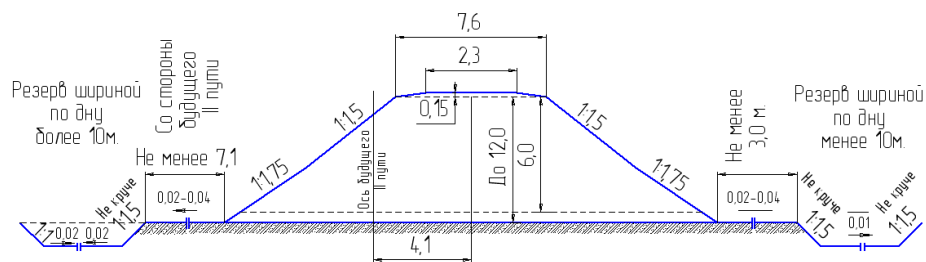
Рис 1 Типовой поперечный профиль земляного полотна: а) – насыпь; б) – выемка.
